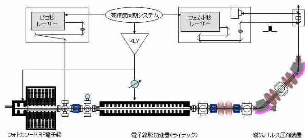
図 2: レーザーフォトカソード RF 電子銃フェムト秒ライナックによるパルスラジオリシス装置
