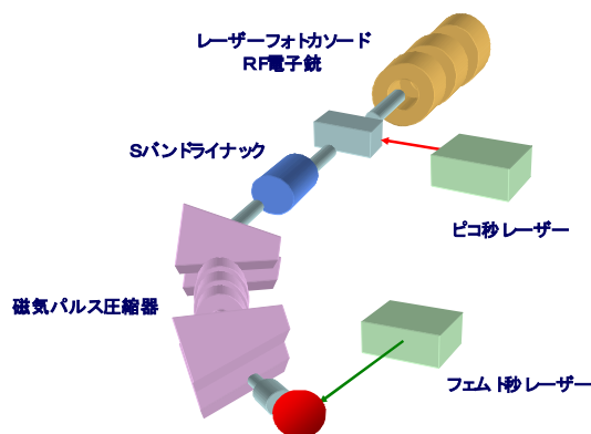
図 1: ナノ空間反応解析のためのフェムト秒・サブピコ秒パルスラジオリシス装置の概念図
