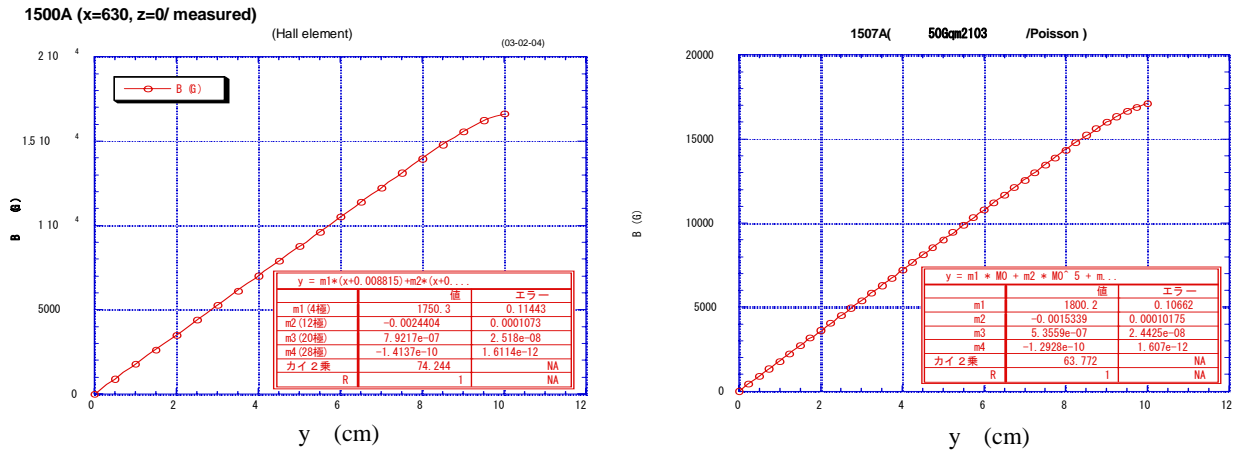
図 8 : 4 極電磁石の横方向磁場分布 (左) 実機 1 号機測定結果 (ホール素子)、(右) POISSON の計算結果
