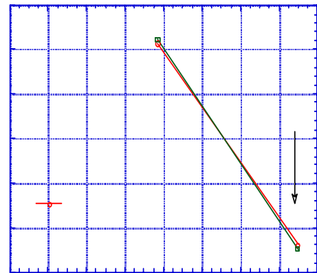
図 10 : 4 極電磁石の有効長の励磁レベル依存性(ホール素子)
