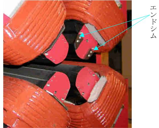
図4 取り付けたエンドシム
