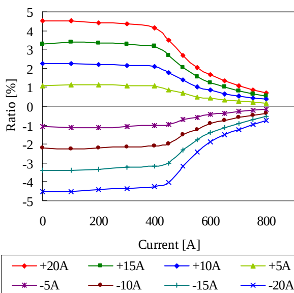
図8 補正コイルによる磁場変化
