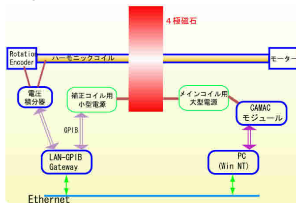
図 2 測定システムの概略
