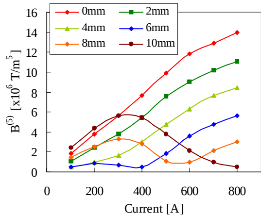
図5 エンドシムの厚さと12極成分の強さ
