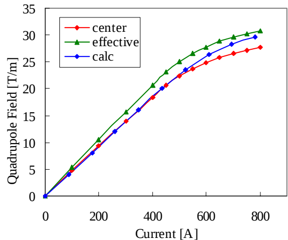
図6 励磁曲線
