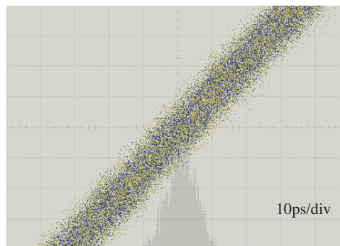
図 7 : 第 5 セクタにおけるマスタートリガーのジッター測定。
