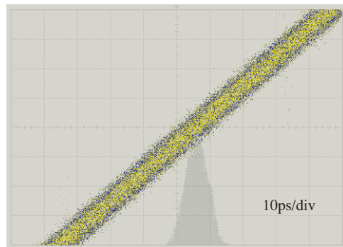
図 4 : メインステーションにおけるマスタートリガーのジッター測定。
