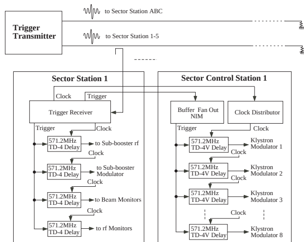
図 6 : セクタステーション及び副制御室におけるトリガー信号分配のブロック図。
