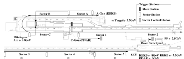
図 1: 入射器におけるトリガーステーションの配置。
