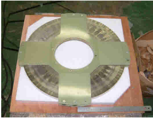
図5 誘導加速空洞用磁性体コア
