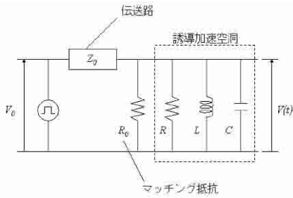
図1 誘導加速装置等価回路
