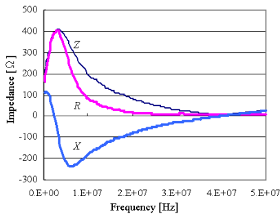
図2 モジュレータからみたインピーダンス
