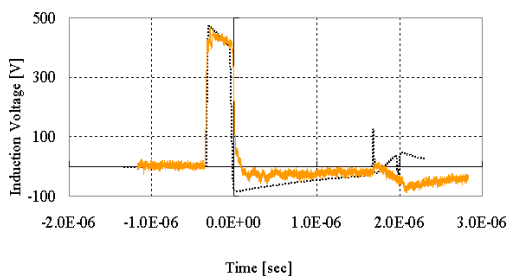
図3 パルス応答に対する測定とシミュレーション
