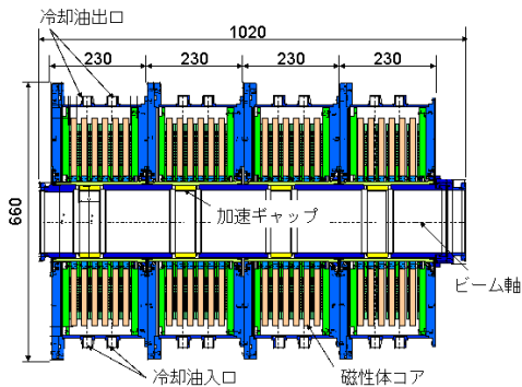
図6 4連加速空洞概観図
